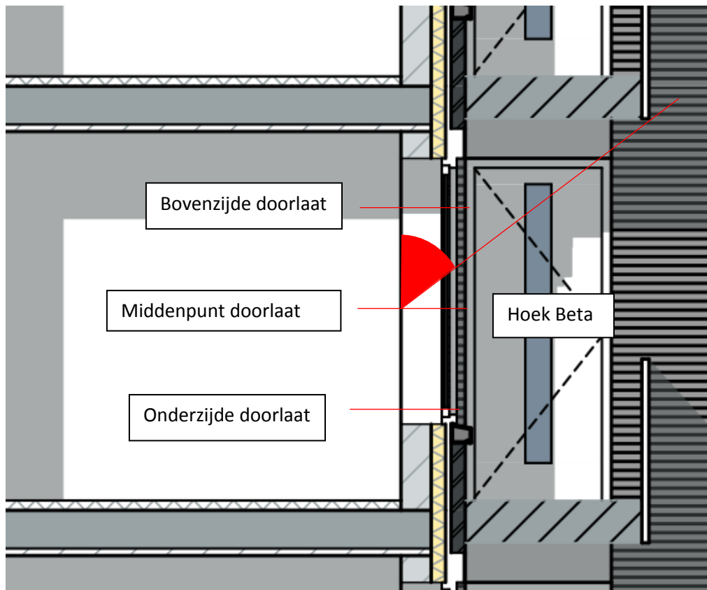
Afbeelding 3: Bepaling hoek Beta met verlaging middenpunt
