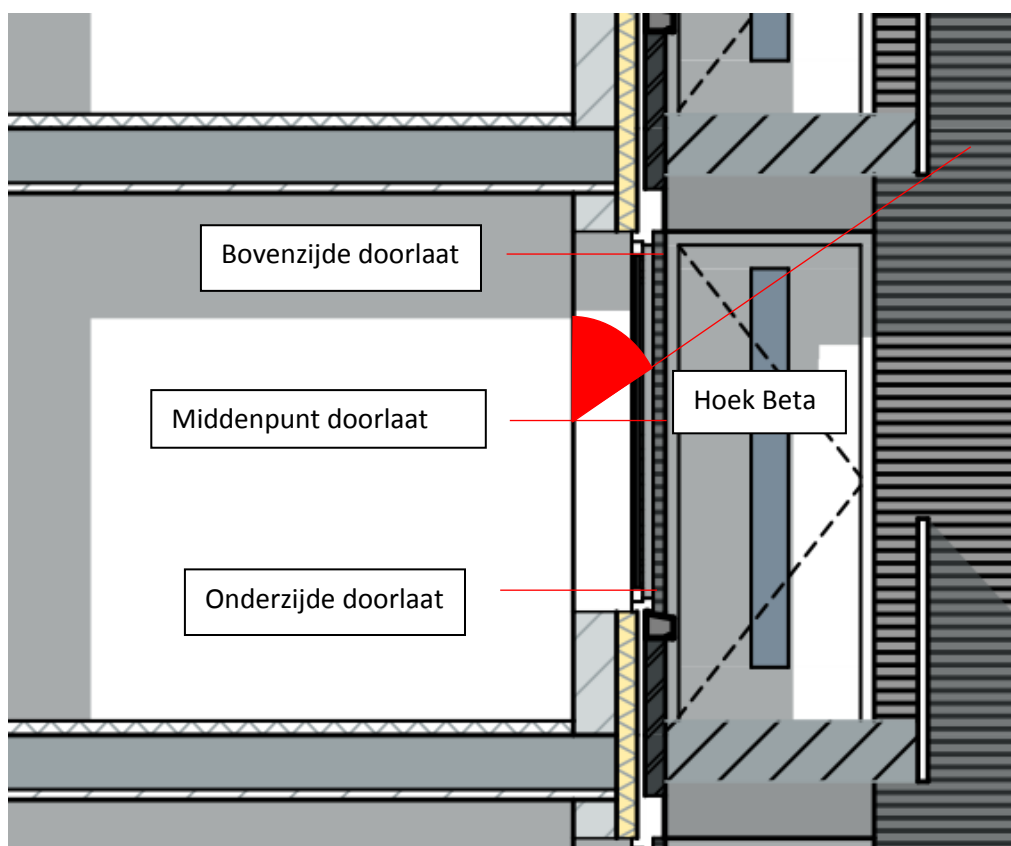
Afbeelding 2: Bepaling hoek Beta zonder aanpassing
